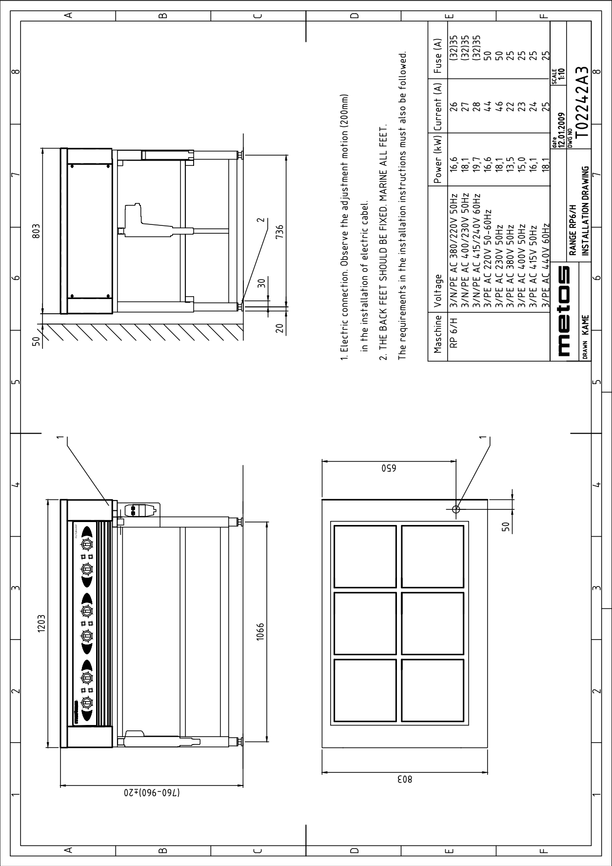
T02242A3 Installationsritning RP6 med höjdjustering
